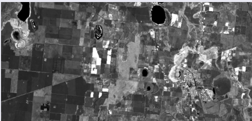
EVI
