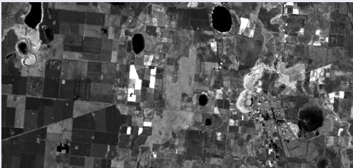
NDVI
